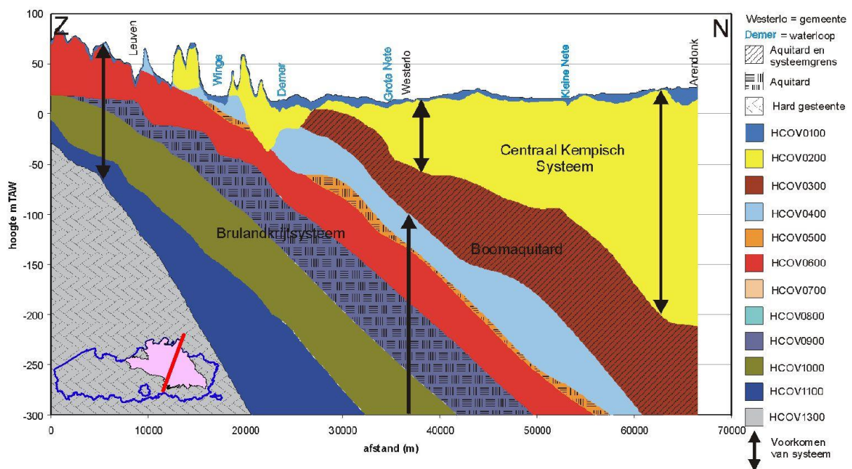
Figuur 2. Zuidwest-noordoost profiel door het Centraal Kempisch Systeem en het Brulandkrijtsysteem.
