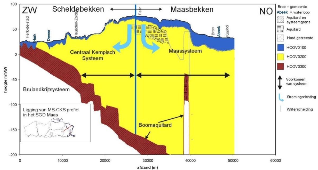
Figuur 1. Zuidwest-noordoost profiel door het Maassysteem en het Centraal Kempisch Systeem.
